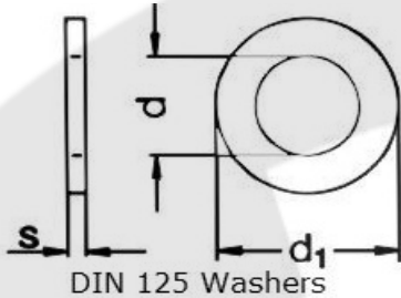
DIN 125 Washers
